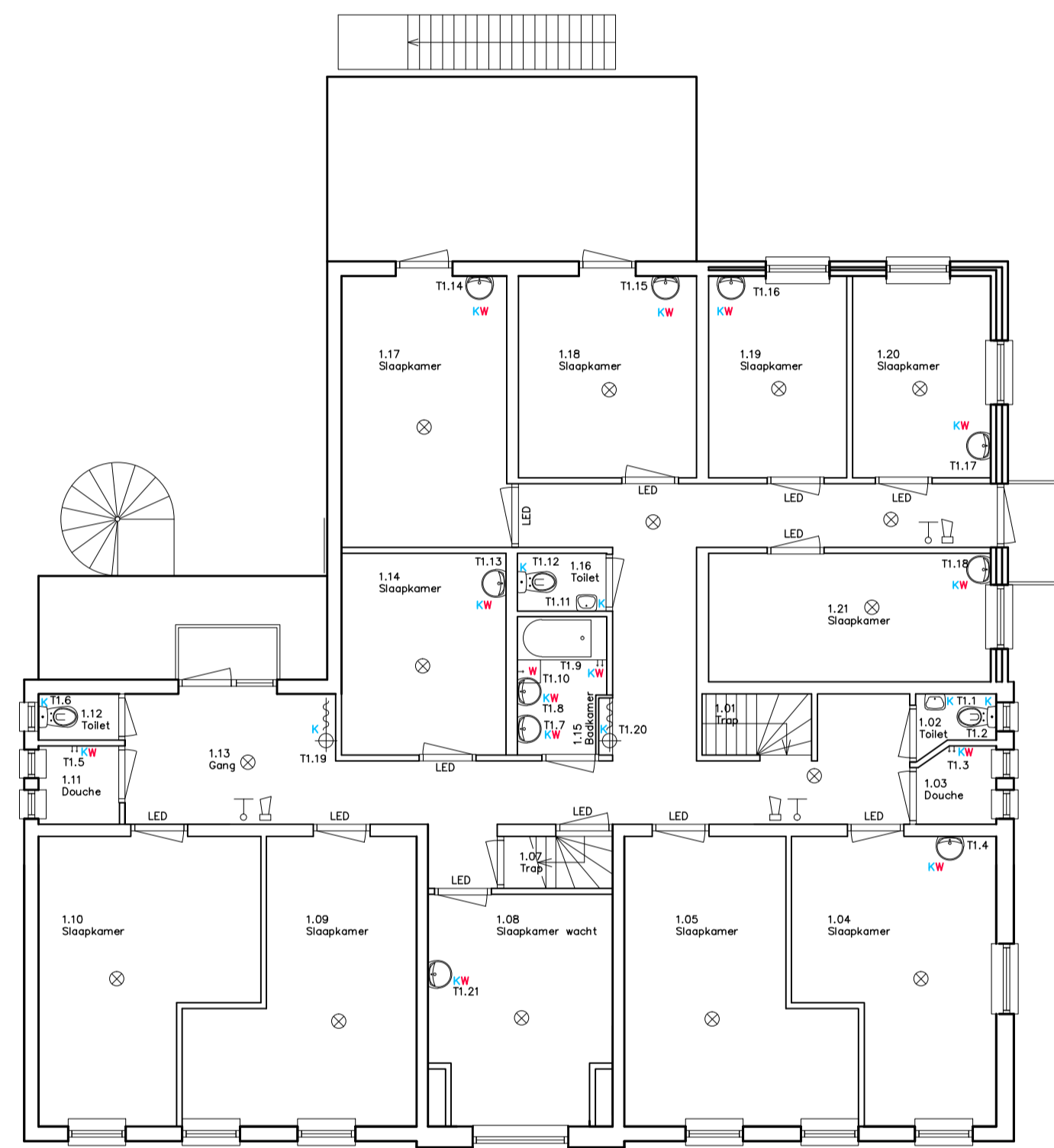
Plattegrond eerste verdieping
